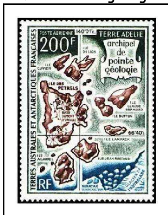
1971 - Pointe géologie
