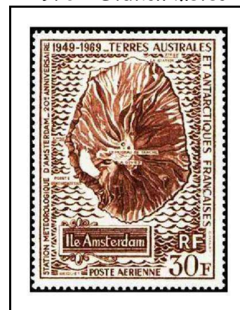
1970 - Station météo
