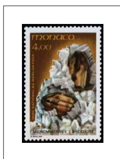
Brookite
